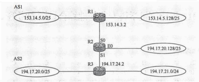
题 47 图 网络拓扑结构
