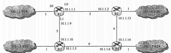
题 42 图 R1 构造的网络拓扑
